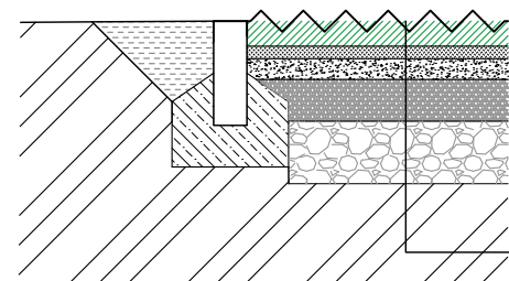
CHARAKTERISTICKÝ REZ M 1:20
